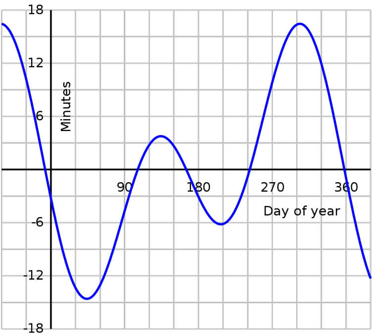
图 3.3: 时差曲线
