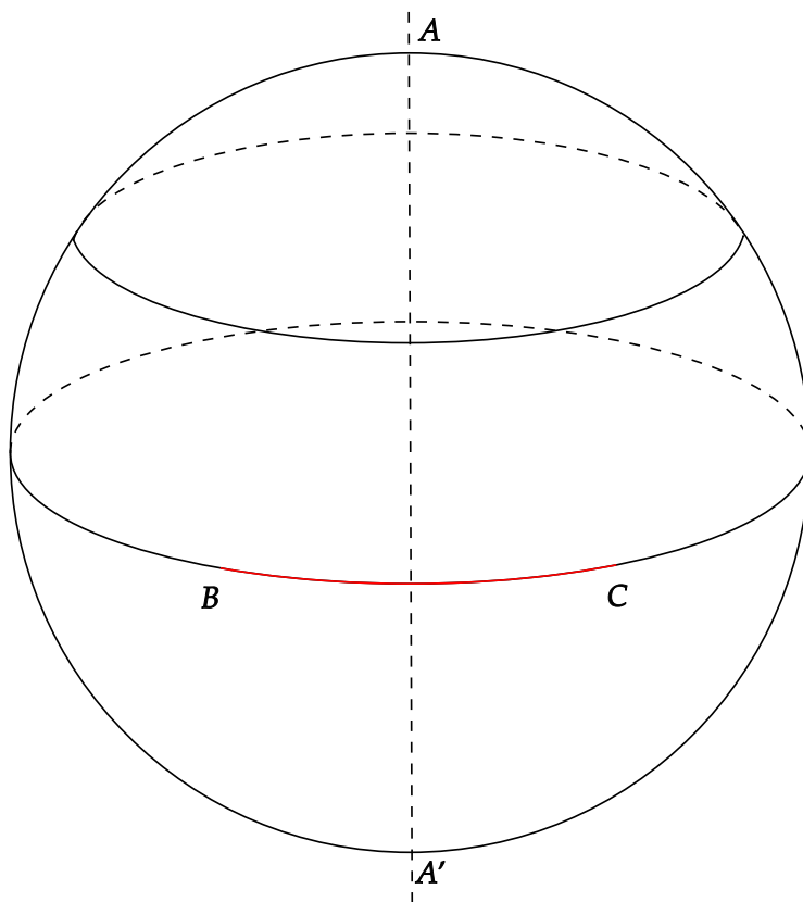
图 3.5: 大圆与小圆
