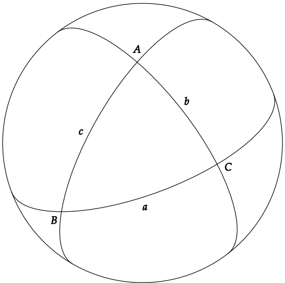
图 3.6: 球面三角形
